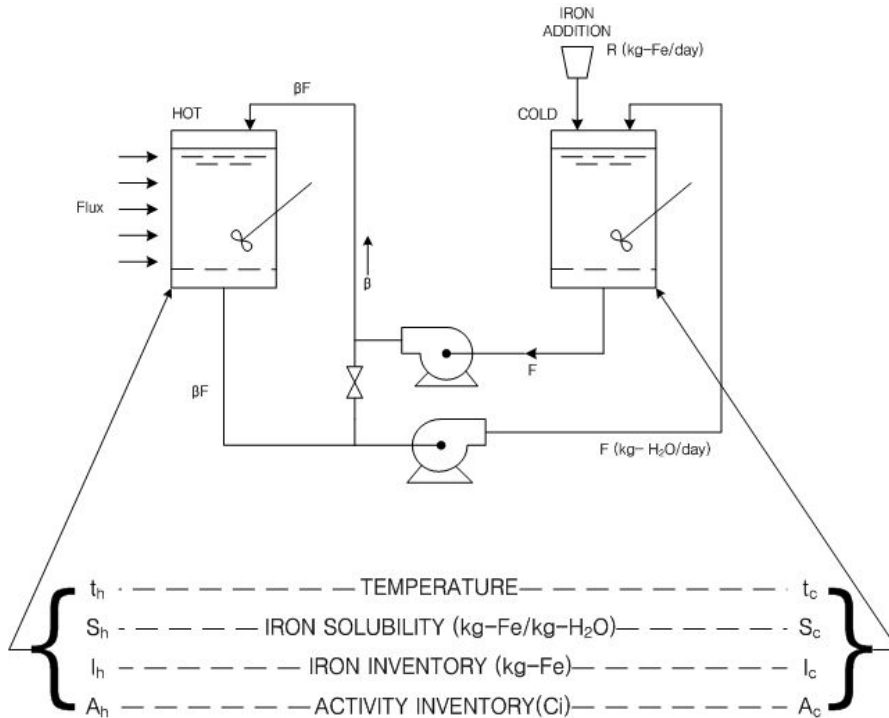
그림 3. CRUDSIM 모델의 전체 개념도[1]
