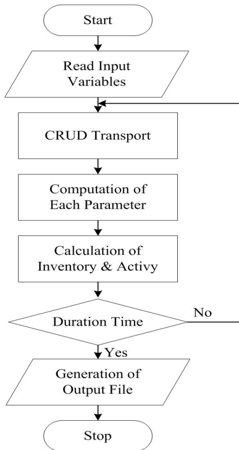
그림 4. CRUDESIM 코드의 계산 과정 순서도[2,4]
