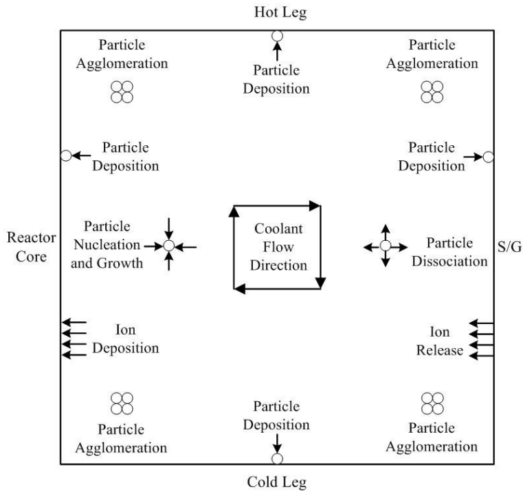
그림 1. 1차 계통내에서의 부식생성물의 이동 메커니즘[1,2,4]
