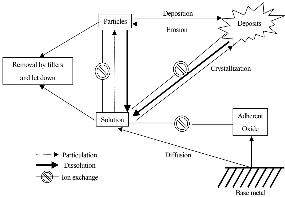
그림 6. PACTOLE 프로그램 계통 모델링[3]
