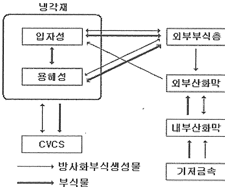
그림 7. ACE 코드의 부식생성물 및 방사화부식생성물 거동 모델[7]
