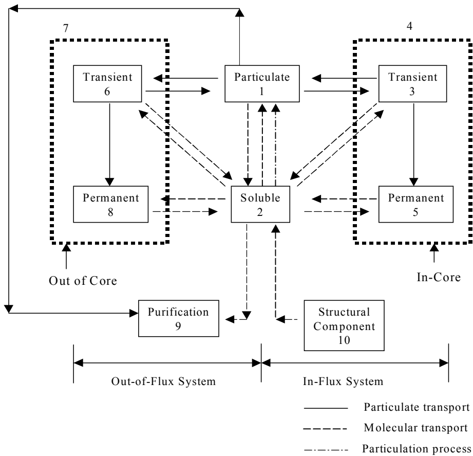
그림 2. CORA 프로그램의 부식생성물 거동 모델링[1]
