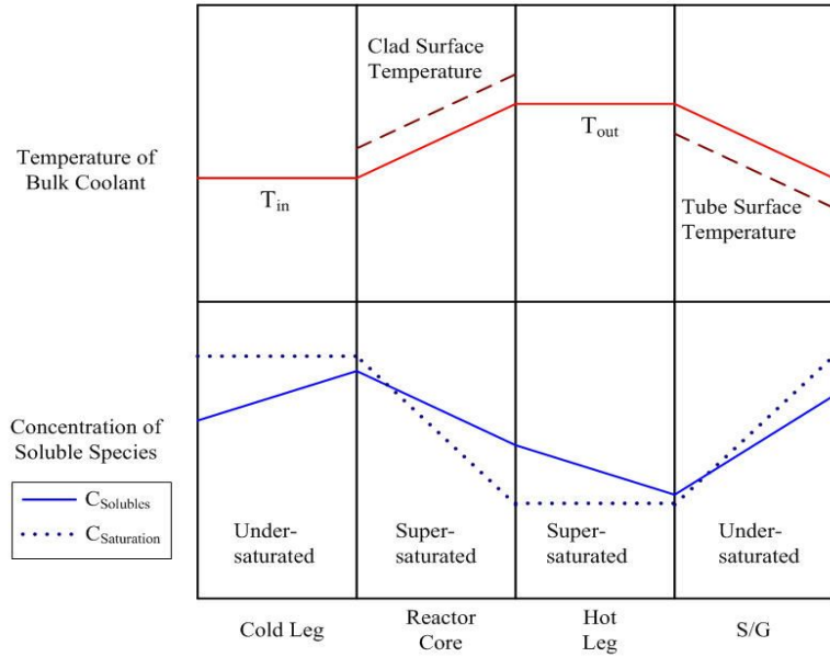
그림 5. 가압경수로 1차 냉각재 계통에서의 냉각재 온도와 용해성[4]
